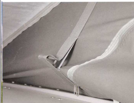
Mécanisme de rabattement du soufflet en tissu
